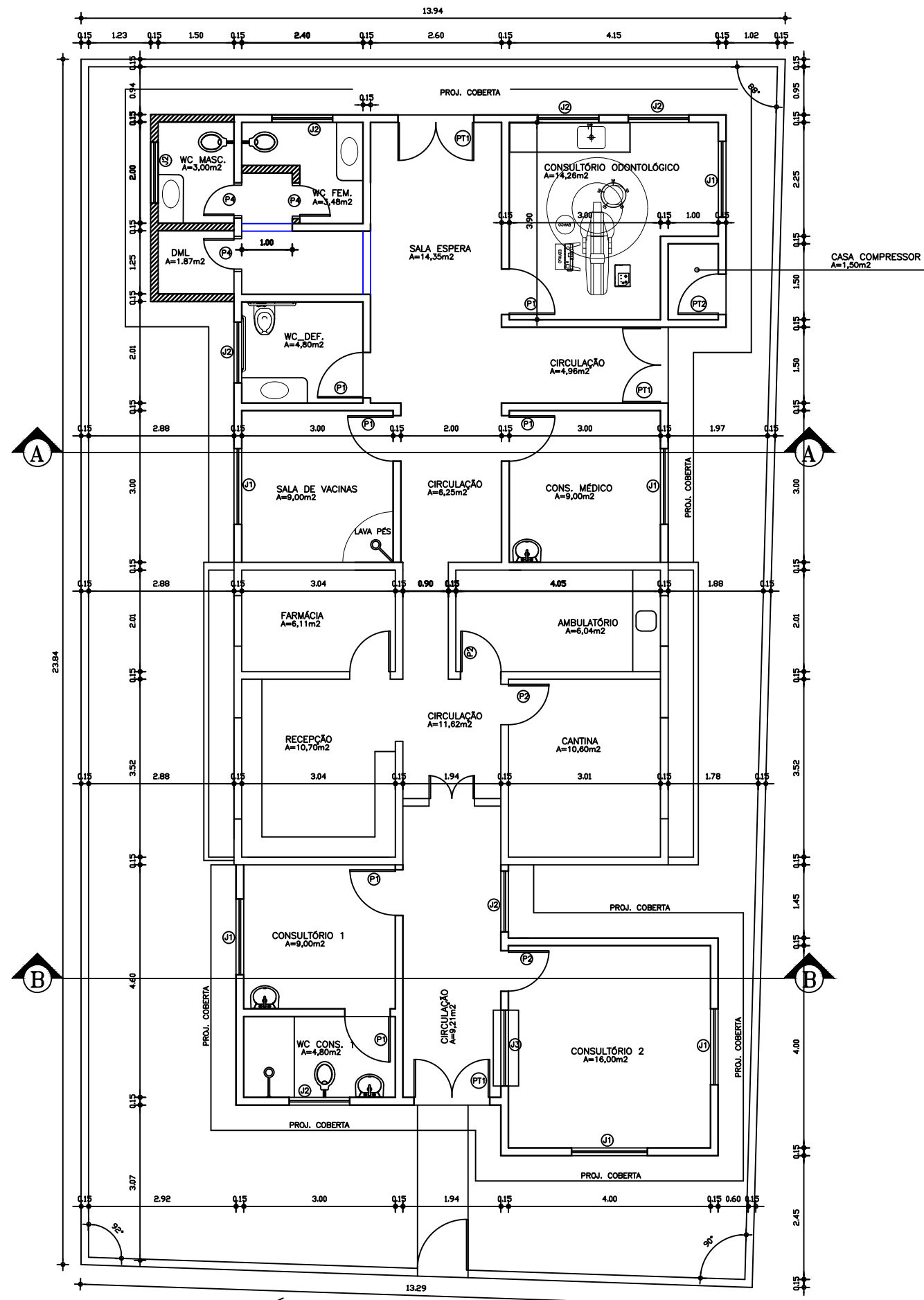
PLANTA BAIXA TÉRREO ESCALA 1/50
