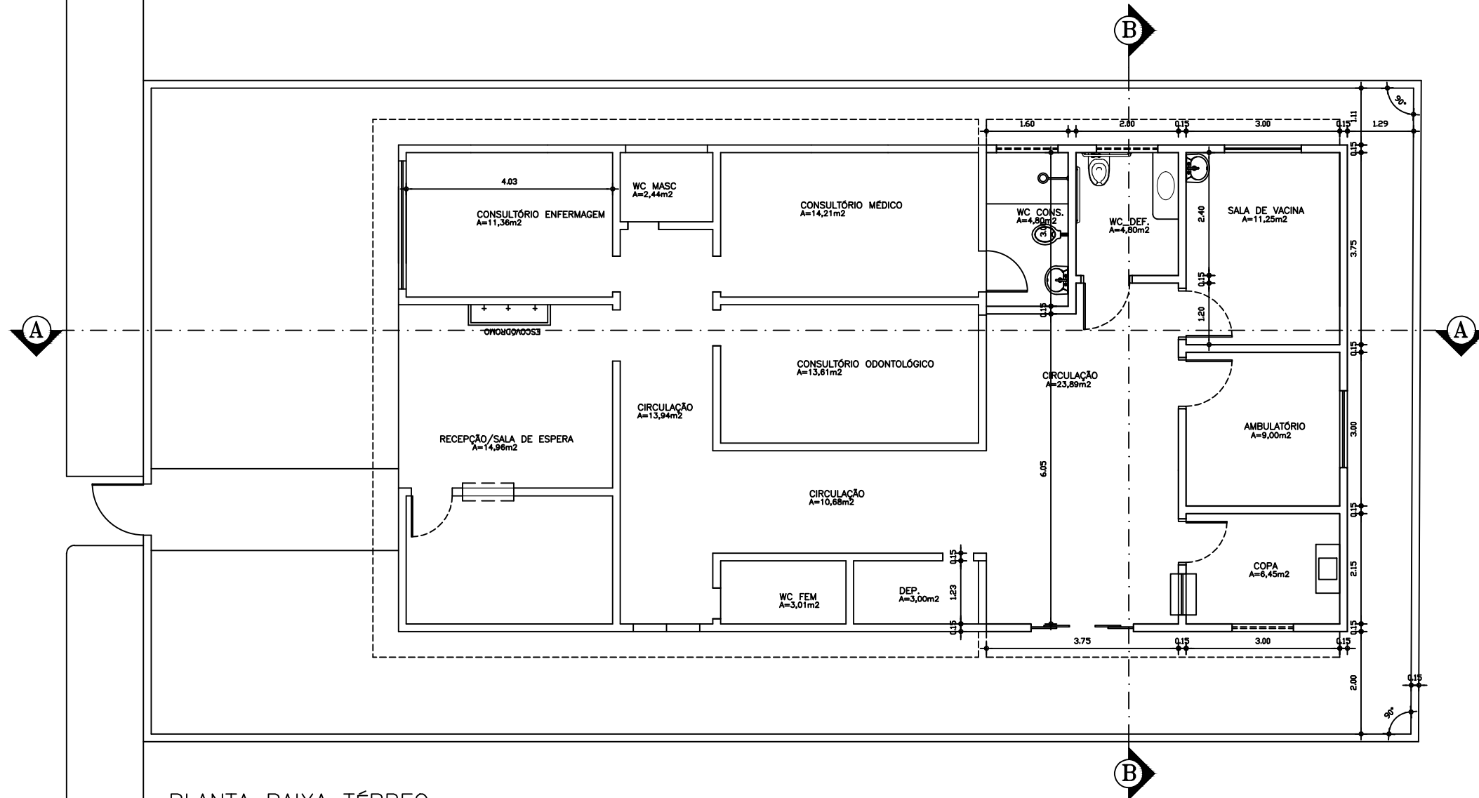
PLANTA BAIXA TÉRREO ESCALA 1/50
