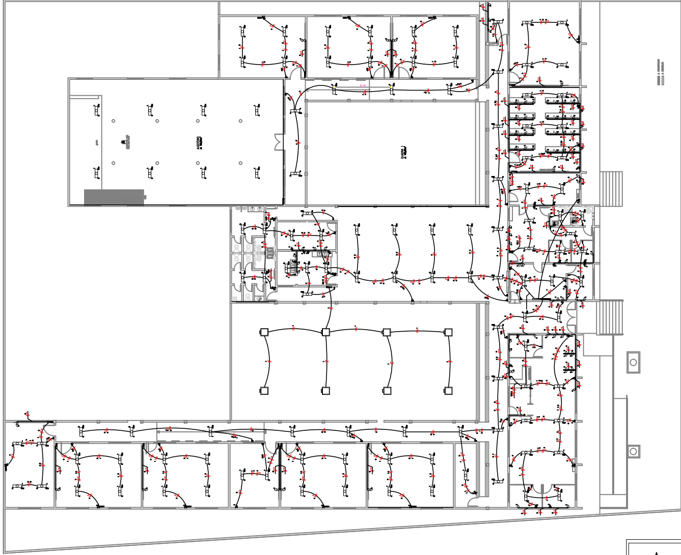
01 PLANTA ELÉTRICA ESCALA — 1 : 200
