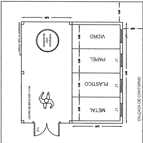
1 PLANTA BAIXA Escala 1/160
