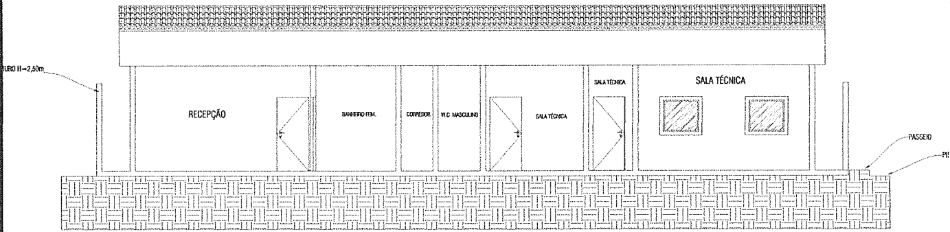
02 CORTE BB ESCALA — 1 : 75
