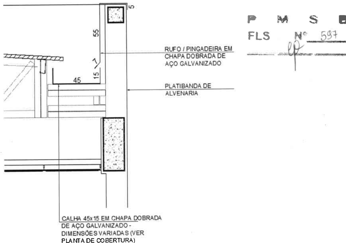
Figura 12 – imagem exemplificativa de detalhe de calha e rufo/pingadeira
