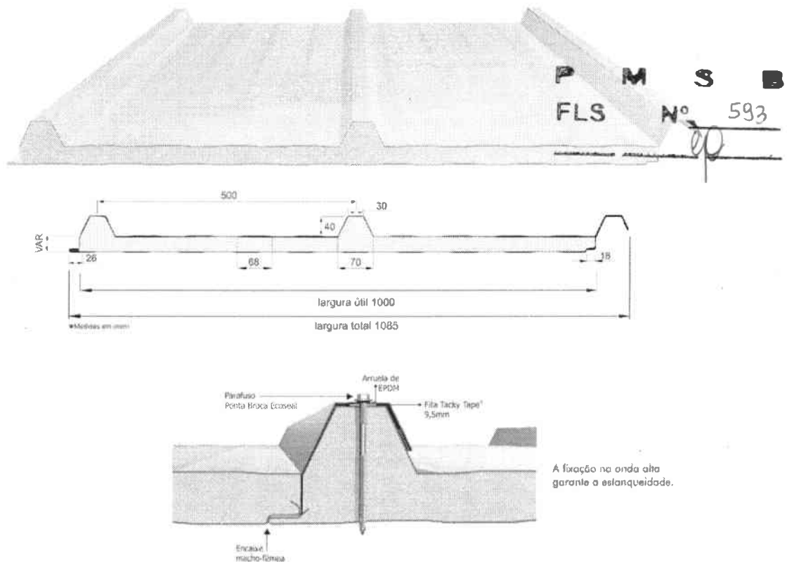
Figura 10 – imagem telha termoacústica
